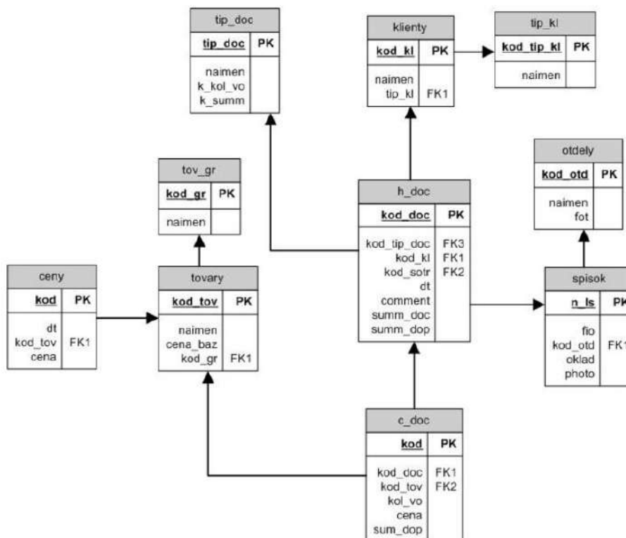
Рисунок 1.1 – Диаграмма базы данных «Склад»
